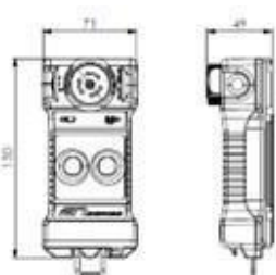
Nadajnik
